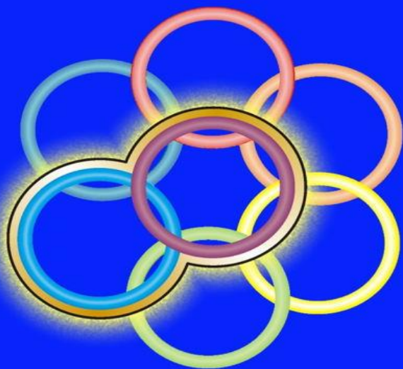
РИСУНОК № 6. ВЫДЕЛЕННЫ КОЛЬЦА, СИМВОЛИЗИРУ- ЮЩИЕ ЭФИРНУЮ И ТЕМПОРАЛЬНУЮ МАТЕРИИ. ЭФИР- НАЯ И ТЕМПОРАЛЬНАЯ МАТЕРИИ ДОМИНИРУЮТ.
