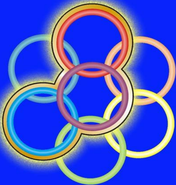
РИСУНОК № 7. МАТЕРИАЛЬНАЯ СИСТЕМА, В КОТОРОЙ ДОМИНИРУЮТ ТРИ ВИДА МАТЕРИИ: ЭФИРНАЯ, ТЕМПОРАЛЬНАЯ И ФИЗИЧЕСКАЯ.
