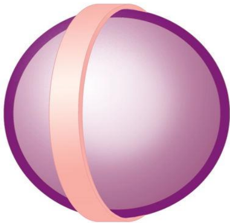
РИСУНОК № 2. КОЛЬЦО И СФЕРА.
