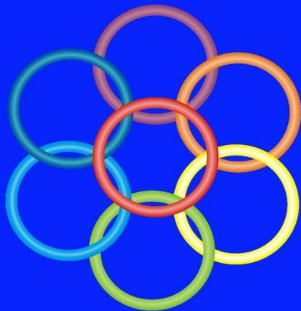
РИСУНОК № 3. ШЕСТЬ КОЛЕЦ ВОКРУГ ОДНОГО. СХЕМА МАТЕРИАЛЬНОЙ СИСТЕМЫ ИЗ СЕМИ ОСНОВНЫХ ВИДОВ МАТЕРИИ. ЦЕНТРАЛЬНАЯ МАТЕРИЯ – ФИЗИЧЕСКАЯ.
