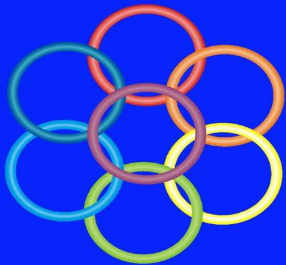
РИСУНОК № 5. ФИОЛЕТОВОЕ КОЛЬЦО В ЦЕНТРЕ. ЭФИРНАЯ МАТЕРИЯ СТАНОВИТСЯ ЦЕНТРАЛЬНОЙ В МАТЕРИАЛЬНОЙ СИСТЕМЕ.
