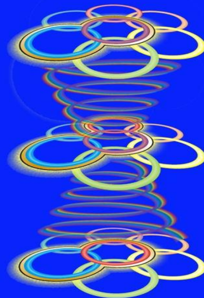
РИСУНОК № 8. ТРИ МАТЕРИАЛЬНЫХ СИСТЕМЫ ВНУТРИ СФЕРЫ КОСМИЧЕСКОЙ ЧЁРНОЙ ДЫРЫ.
