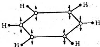
Рис. 2. Схема молекулы бензола
