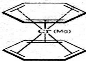
Рис. 3. Схема молекулы дихромбензола
